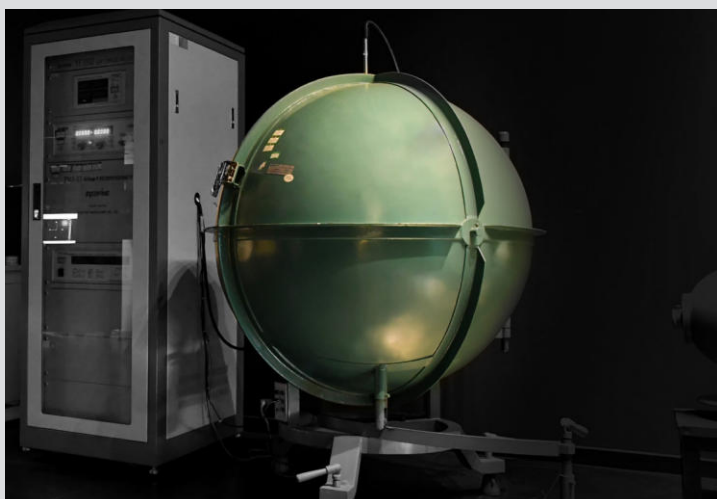
Ulbricht-Kugel
